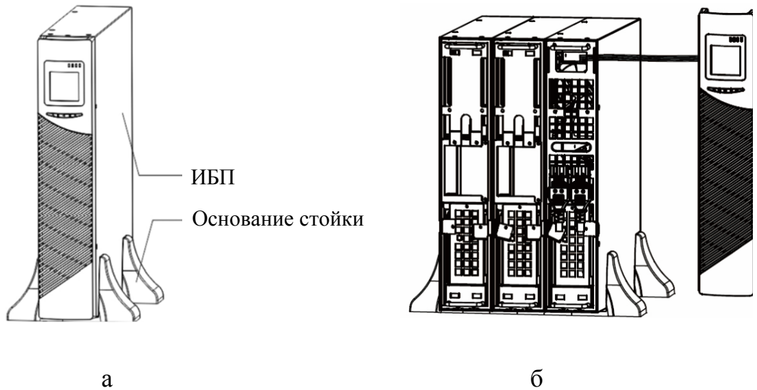
Рисунок 2.7 – Установка блока ИБП и блоков АКБ
