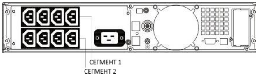
Рисунок 1.7 – ИБП напольно-стоечного исполнения СИПБ1,5КА.9-11, СИПБ2КА.9-11, вид задней панели
