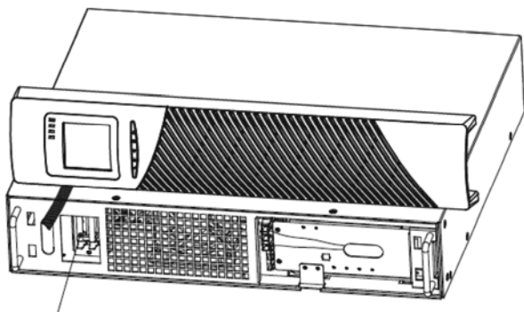
Место установки плавкого предохранителя в блоке ИБП
