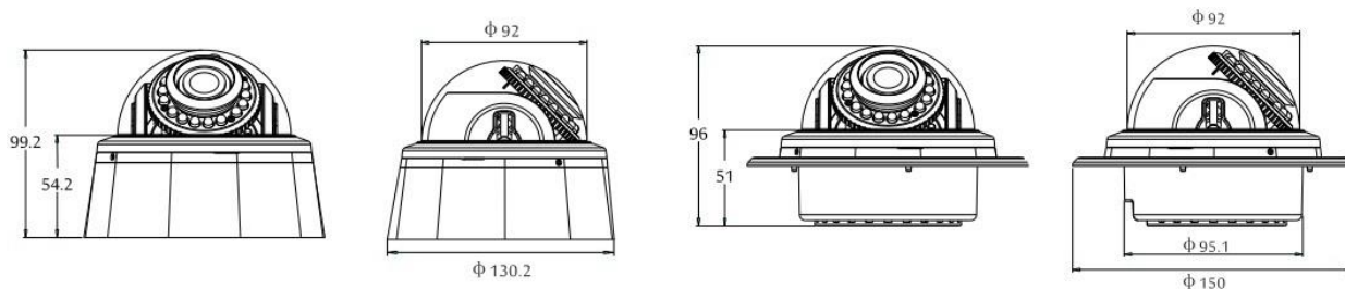
Габариты при накладном монтаже: 130.2 (Ø) x 99.2 мм (В)
