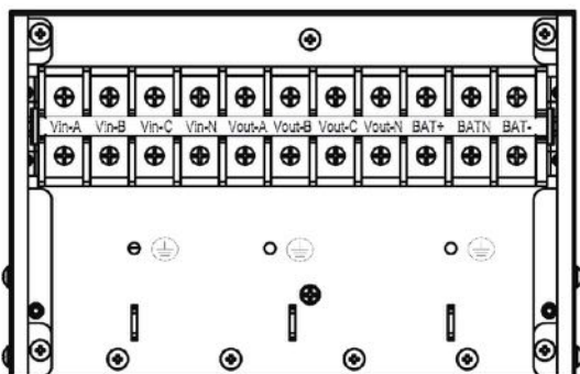
Рис. 6: 10-20 кВА
