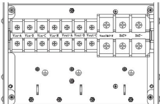
Рис. 7: 30-40 кВА:
